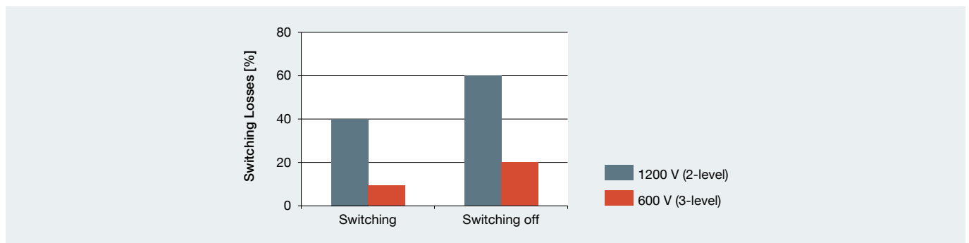
Fig. 3 - Perdas de comutação para IGBTs de 1200 V e 600 V.
