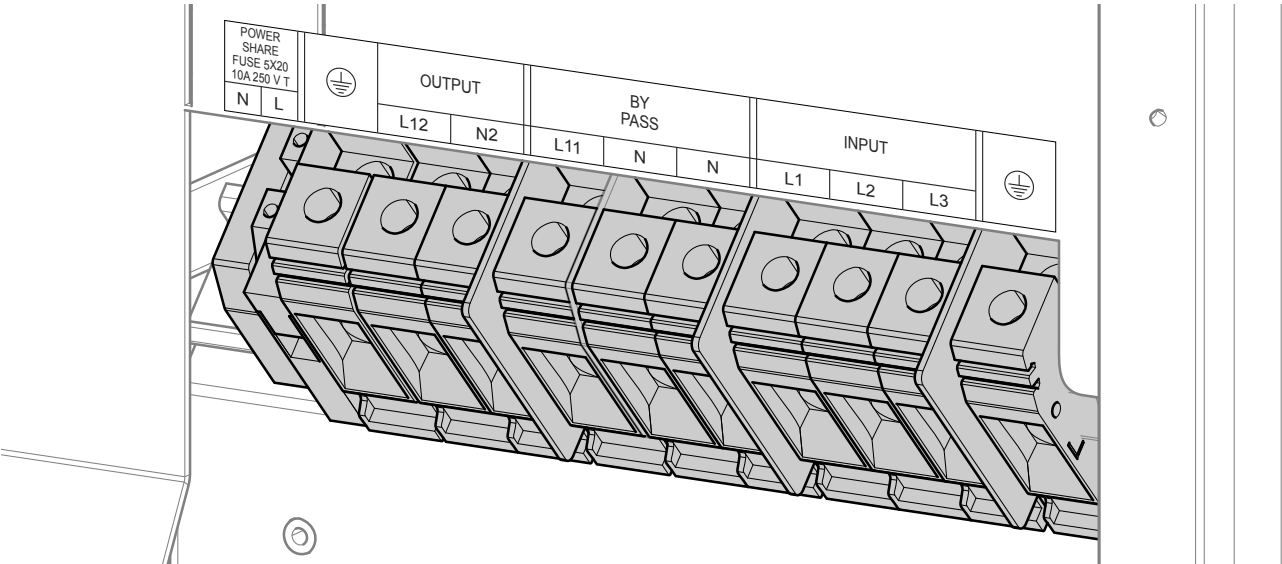
Disposição dos blocos terminais
