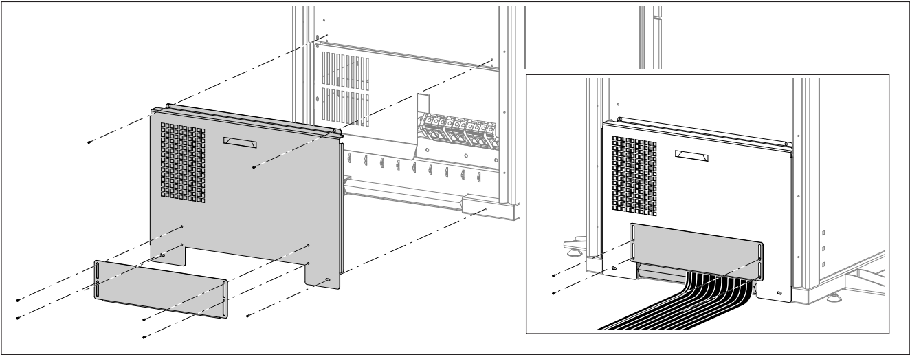
Disposição dos blocos terminais
