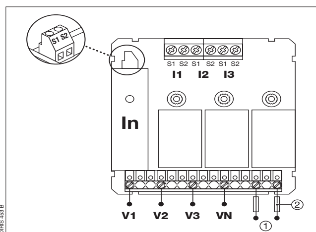
DIRIS A-41
