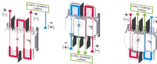
接线方式1
