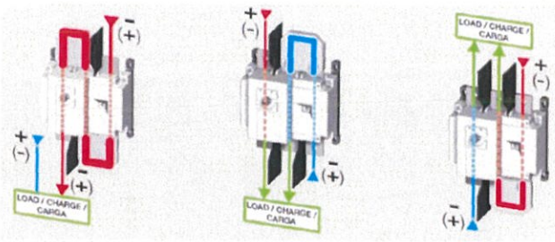
接线方式1
